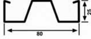
GALVANİZ M PROFİLLERİ
