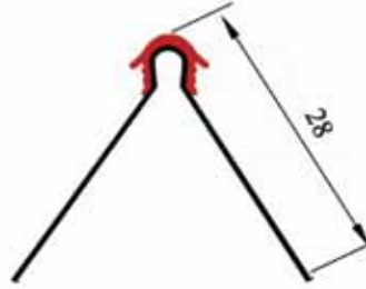
PVC SIRTLI KARE DELİKLİ SIVA KÖŞE PROFİLİ
