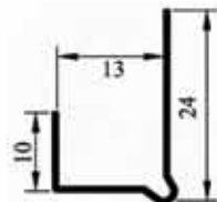
ALÇIPAN DETAY U BİTİM PROFİLLERİ
