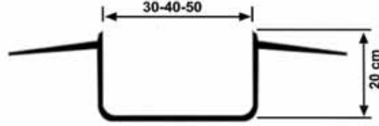
PVC FUGA PROFİLLERİ Pvc Seam Profiles пвх профили для швов
