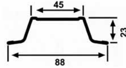
GALVANİZ N PROFİLLERİ
