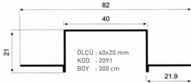
40 mm Alüminyum Fuga
