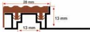
13 mm PVC Bantlı Basamak Profili
