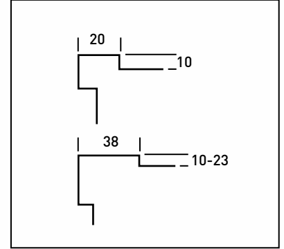
S.S. KÖŞE BİTİŞ PROFİLİ
