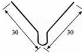
SIVA KÖŞE PROFİLLERİ 30x30
