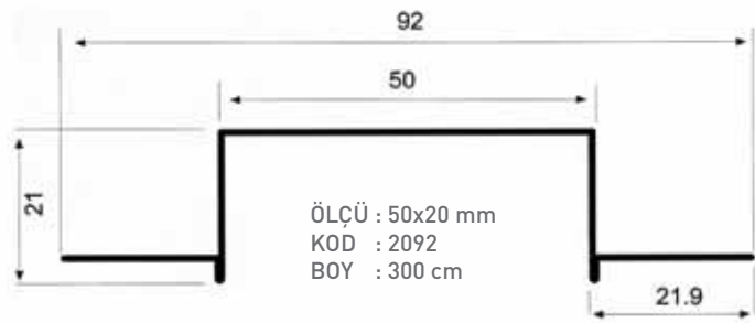
50 mm Alüminyum Fuga
